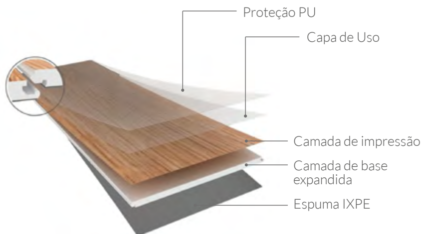
Figura 3. Camadas do revestimento vinílico heterogêneo AUTOPORTANTE
