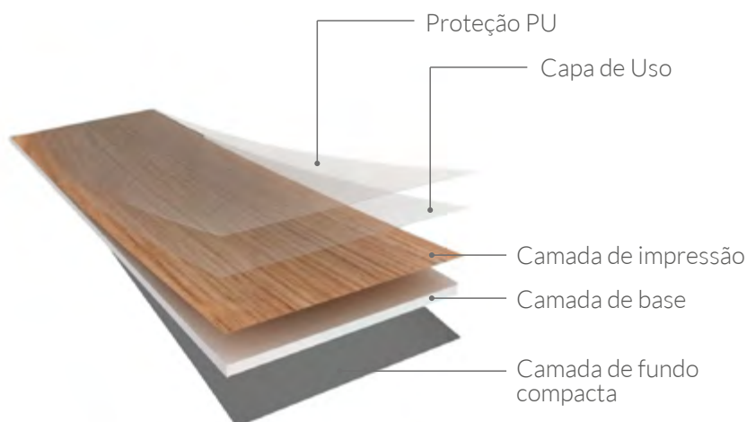
Figura 1. Camadas do revestimento vinílico heterogêneo LVT
