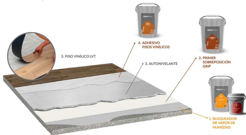
Figura 4. Etapas del proceso de utilización de insumos, contrapiso (cemento o cerámica) térreo
