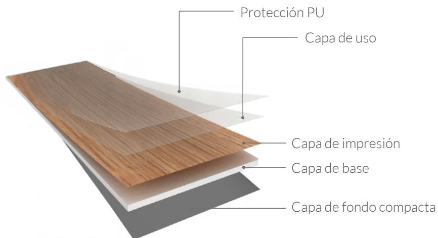
Figura 1. Capas del revestimiento vinílico heterogéneo LVT
