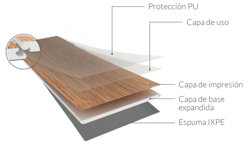
Figura 3. Capas del revestimiento vinílico heterogéneo AUTOPORTANTE
